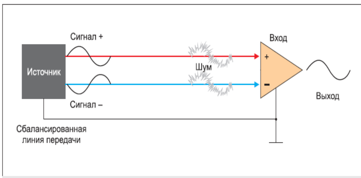
Рис. 2. Балансный сигнал
